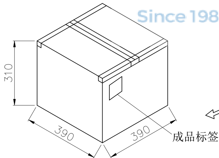
⑤ 外箱封箱示意图
