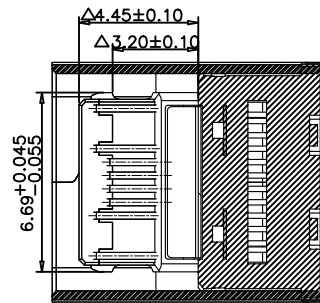
截面B-B
