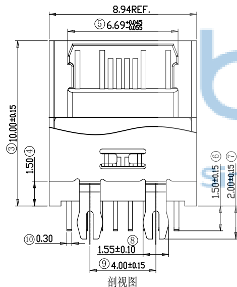
剖视图
