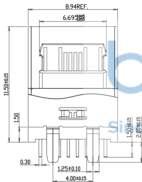
剖视图
