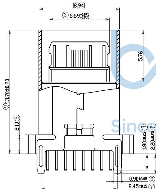
剖视图
