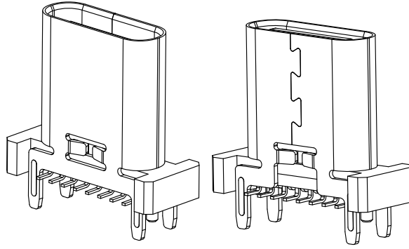
剖视图
