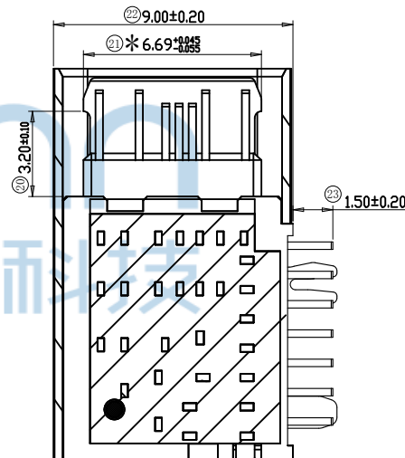
A-A 剖视图
