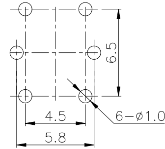
P.C.B LAYOUT
