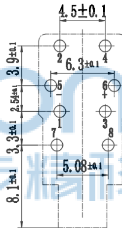
元件面孔位图
