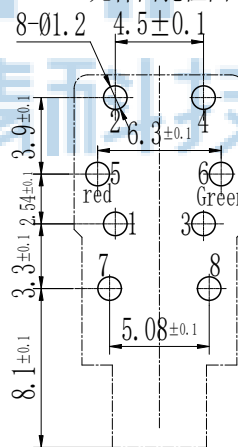
元件面孔位图
