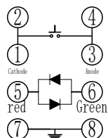
电原理图
