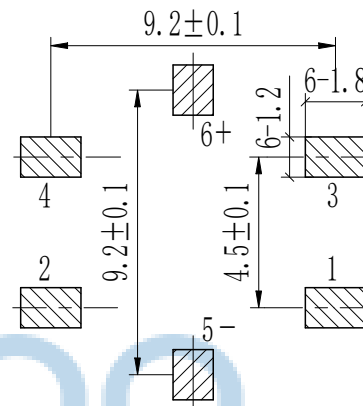
元件面孔位图
