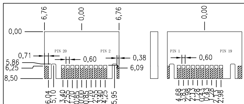
PCB 标示图
