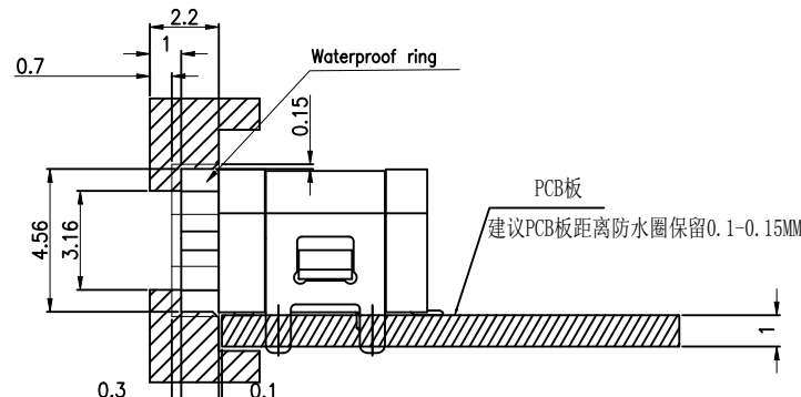
方型圈组装防水示意图
