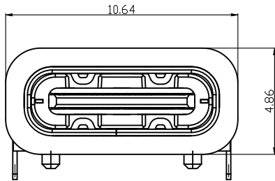
带防水圈示意图
