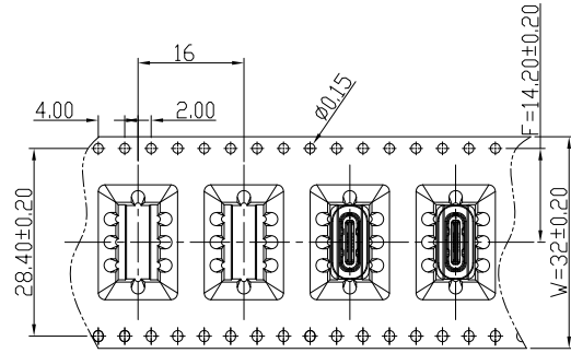
① 产品入载带示意图
