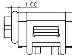
加防水圈示意图
