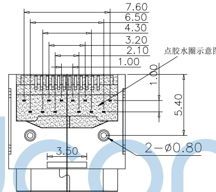
加防水圈示意图
