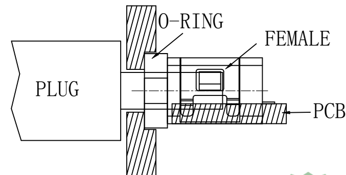
组装面板防水示意图
