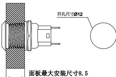
安装视图
