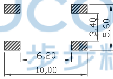
PCB. 焊接图
