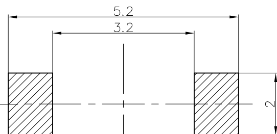
安装参考图
