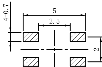
安装参考图
