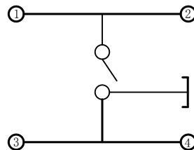
原理图
