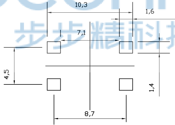
安装尺寸
