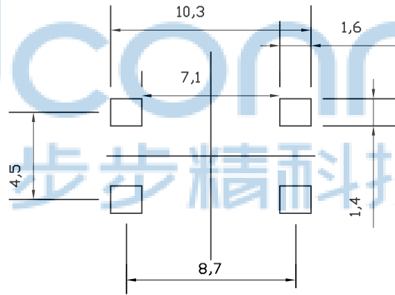
安装尺寸
