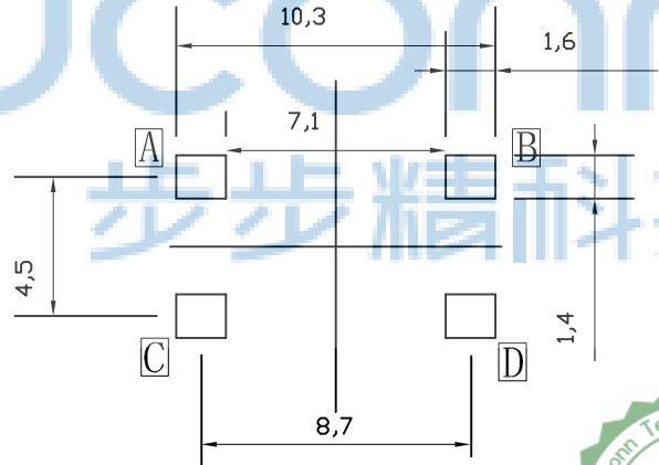
安装尺寸
