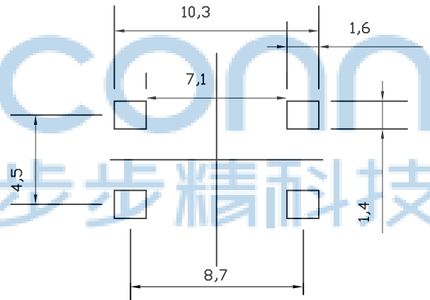
安装尺寸
