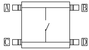
电器原理图
