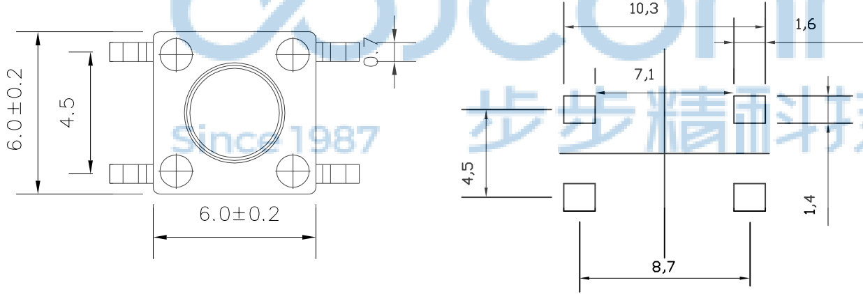
安装尺寸
