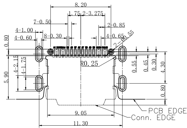
RECOMMENDED PCB LAYOUT TOLERANCE: ±0.05 (建议使用刷钢板厚度0.12mm)
