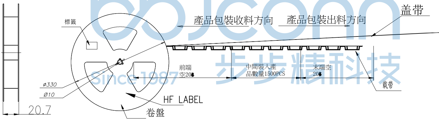
图示(二) 圆盘包装
