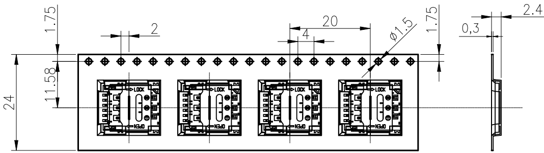
图示(一) 载带
