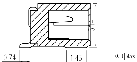
截面 A-A
