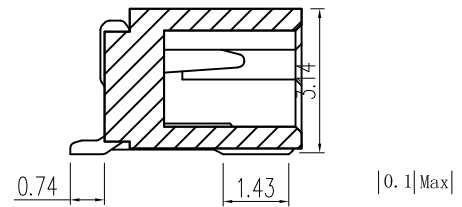
截面 A-A
