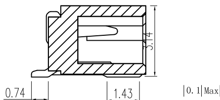
截面 A-A
