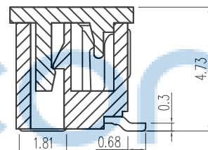
截面 A-A
