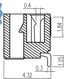
截面 A-A
