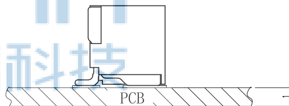
截面 A-A
