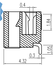
截面 A-A
