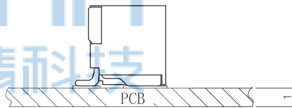
截面 A-A
