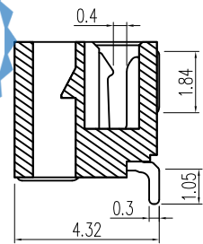
截面 A-A
