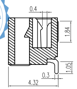
截面 A-A
