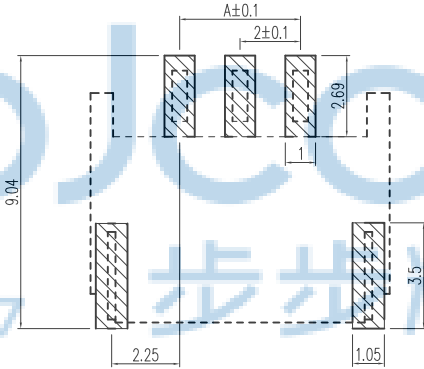
印制线路板
