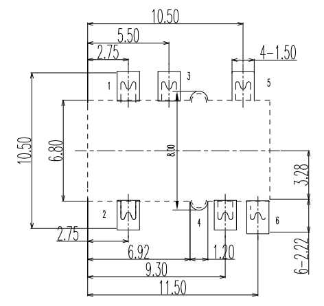
P.C.B LAYOUT TOP VIEW 反贴
