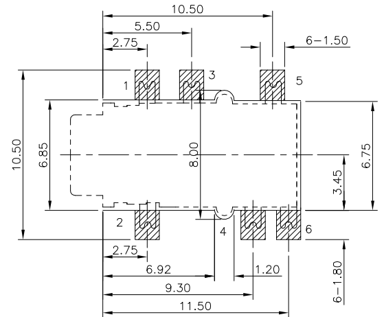
P.C.B LAYOUT TOP VIEW 反贴
